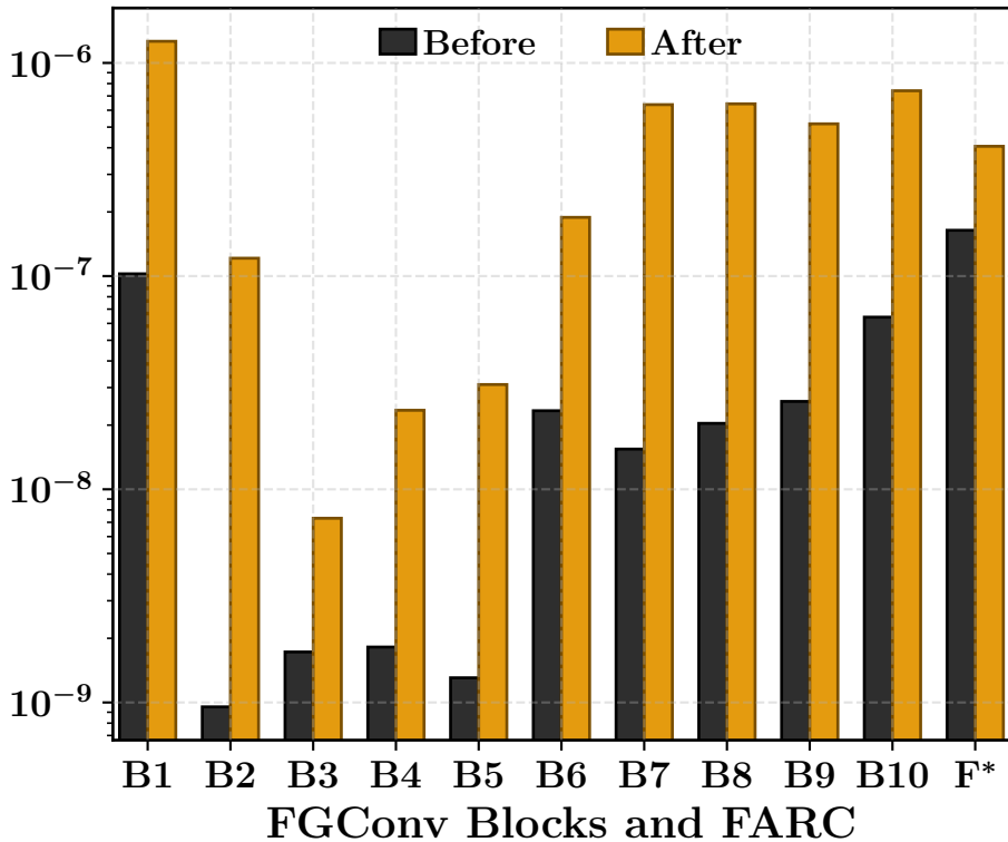
Gradient Variance
